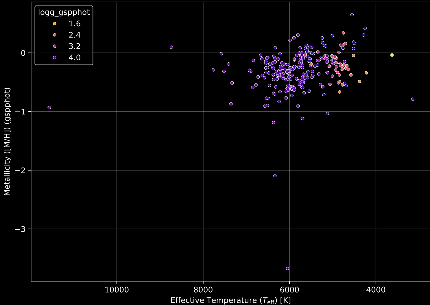
GALAH DR4 Field: [7132] Stellar Population Parameters (n= 259)
