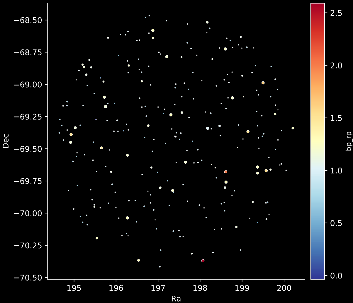
GALAH DR4 Field: [7132] Stars: 259
